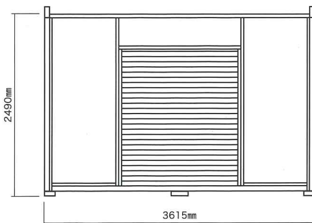
南側立面図
