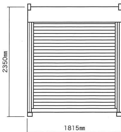
南側立面図
